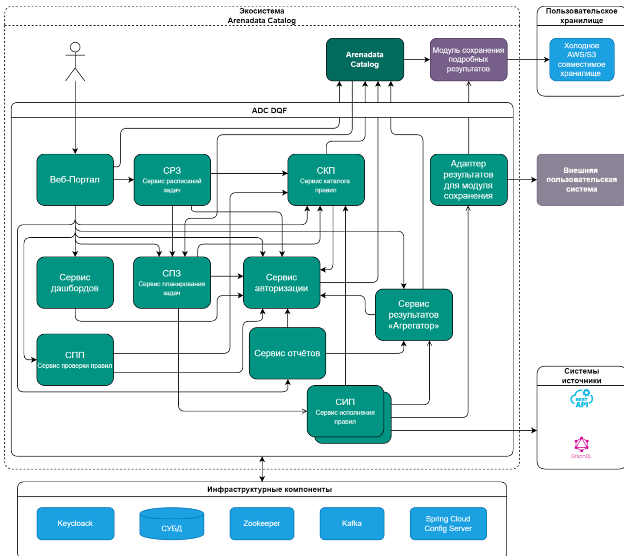
Рисунок 1. Архитектурная схема ADC.DQF.
